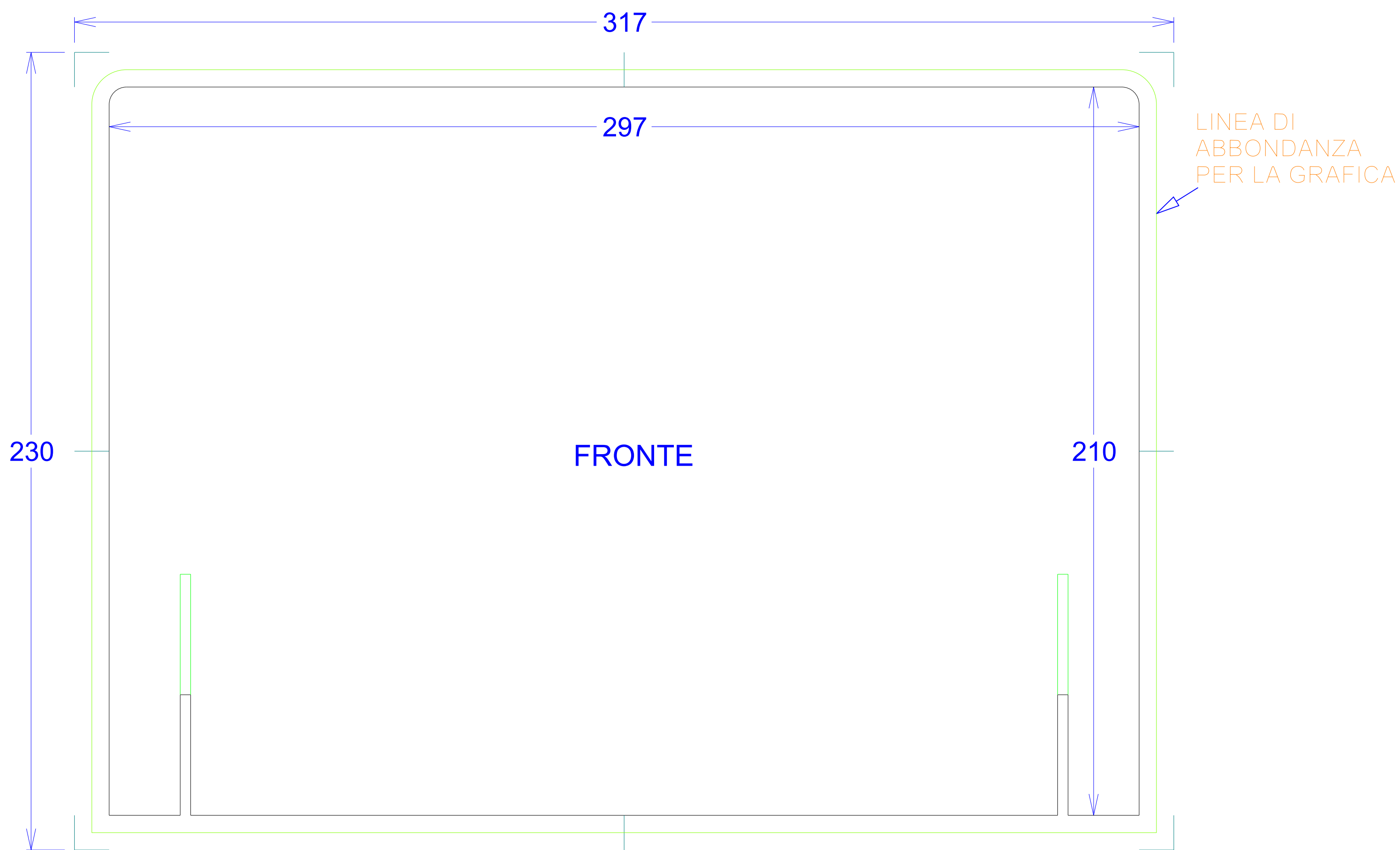
PINZA LATO STAMPA COD. 300_302_3044-01_DIS1
